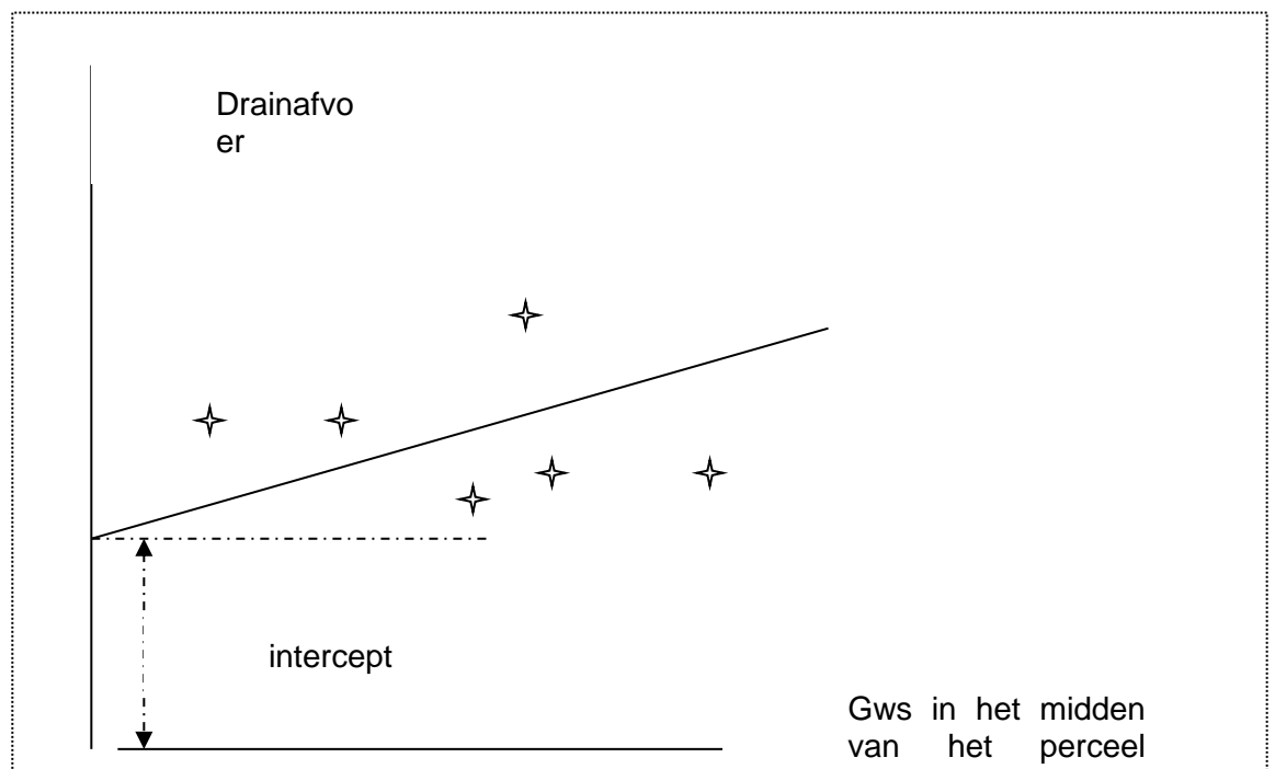
Afb.4: Kengetallen voor drain functioneren (relatie tussen de drainafvoer en de grondwaterstand (gws))
